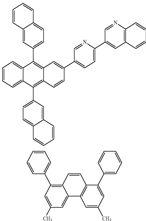
BCP
