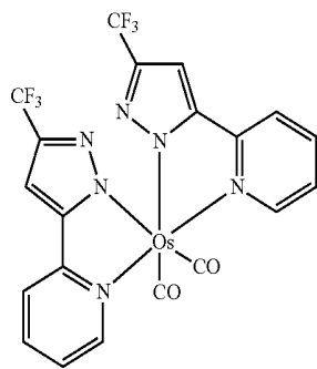
OS(fppz) 2 (CO) 2
